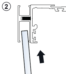
Deckenmontage
