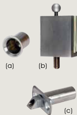
Feststeller FS 01 Bestehend aus: einer Bodenhülse (a), einem Feststeller (b), einem Schnapper (c)
