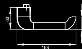
Kent - EPL 96 LH in Edelstahl matt mit Leder hellbraun, auf runder Plan Design Rosette
