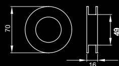
Schiebetürmuschel für Glastür EZ1706 GS – EZ1706 GSH (verschraubbar) Bohrdurchmesser im Glas: 50 mm, TS: 8-11 mm Farbe: Edelstahl matt
