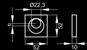
Schutzrosette – ESR 400 Q KS
