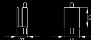
Feststellriegel – EGF 100 mit Bodenhülse, für Glasstärke 8 -10 mm Farbe: Edelstahl matt
