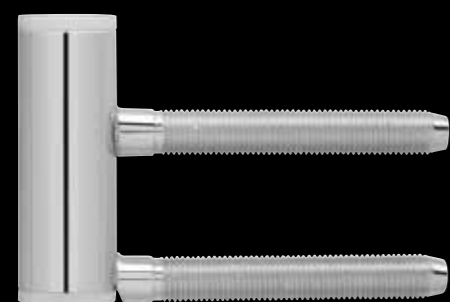
Rahmentteile – EGB 3 V 4400 WF für Holzzargen, Höhe: 48,5 mm Farbe: Stahl verzinkt
