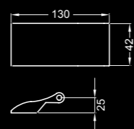
Glastürband 2-teilig – EGB 102 Farbe: Edelstahl matt
